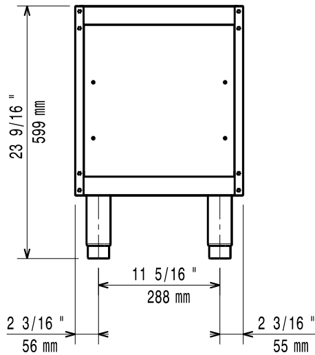
Oldalnézet
